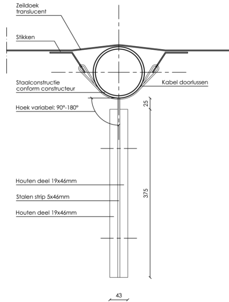
Horizontaal Principedetail Gevel
